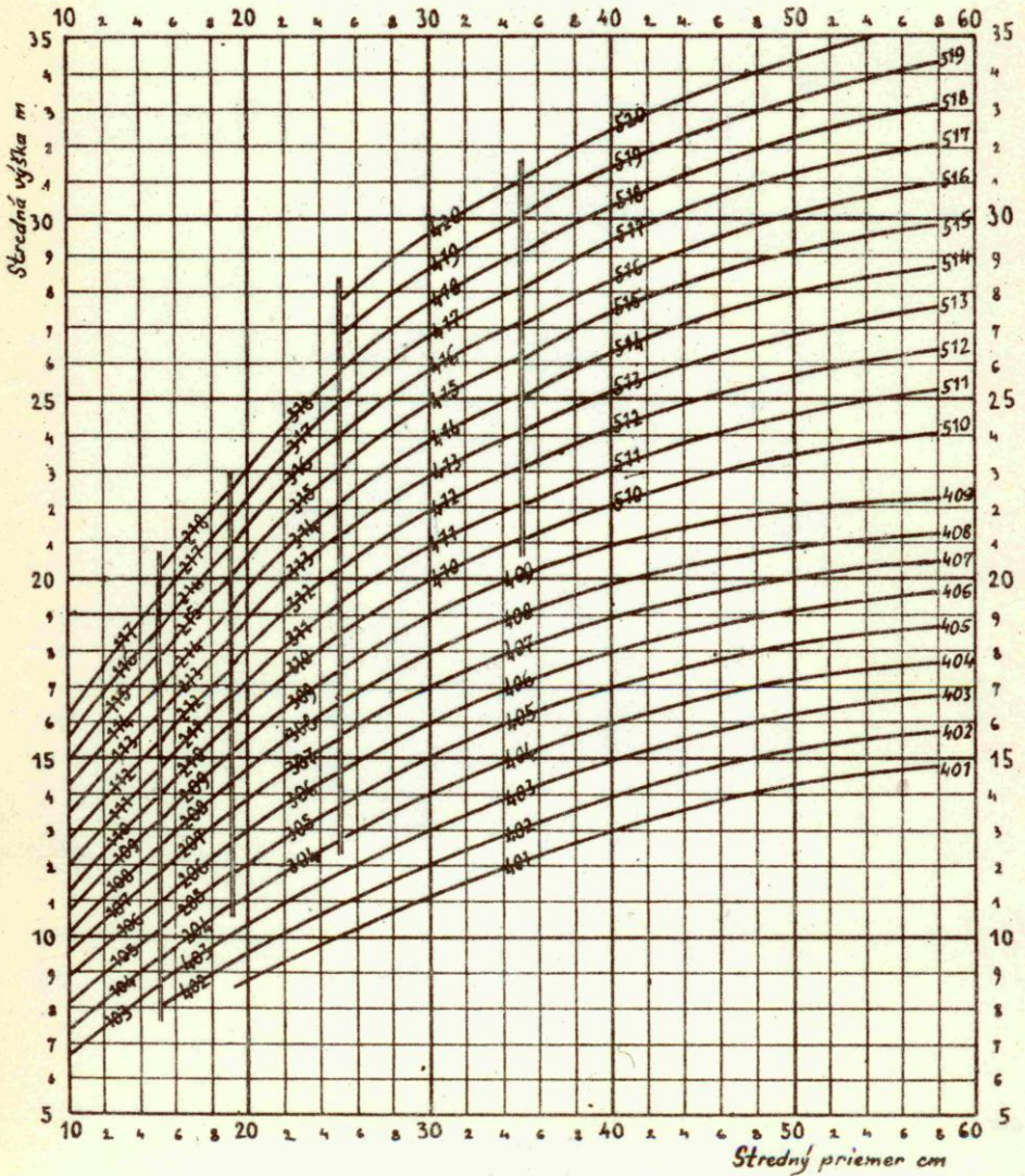
Grafikon pre určenie čísla JOK
