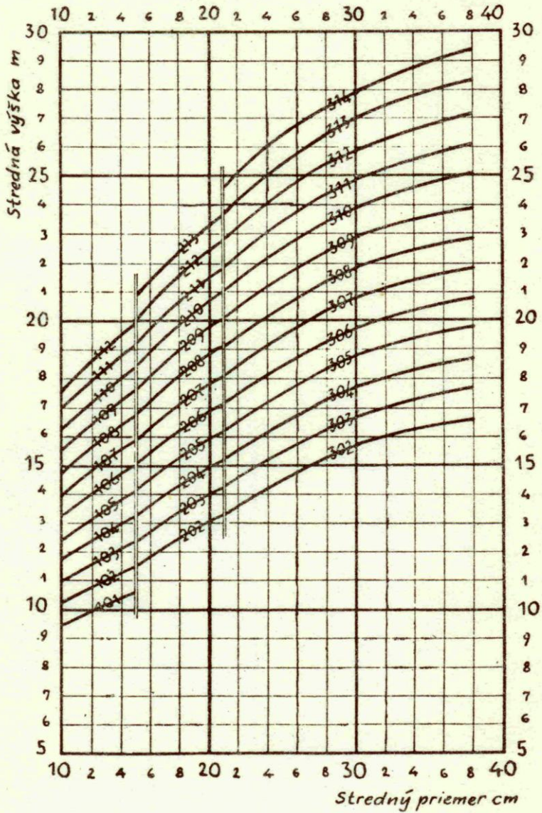
Grafikon pre určenie čísla JOK
