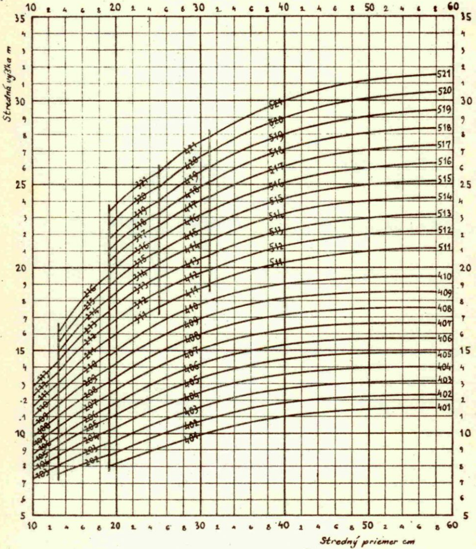
Grafikon pre určenie čísla JOK
