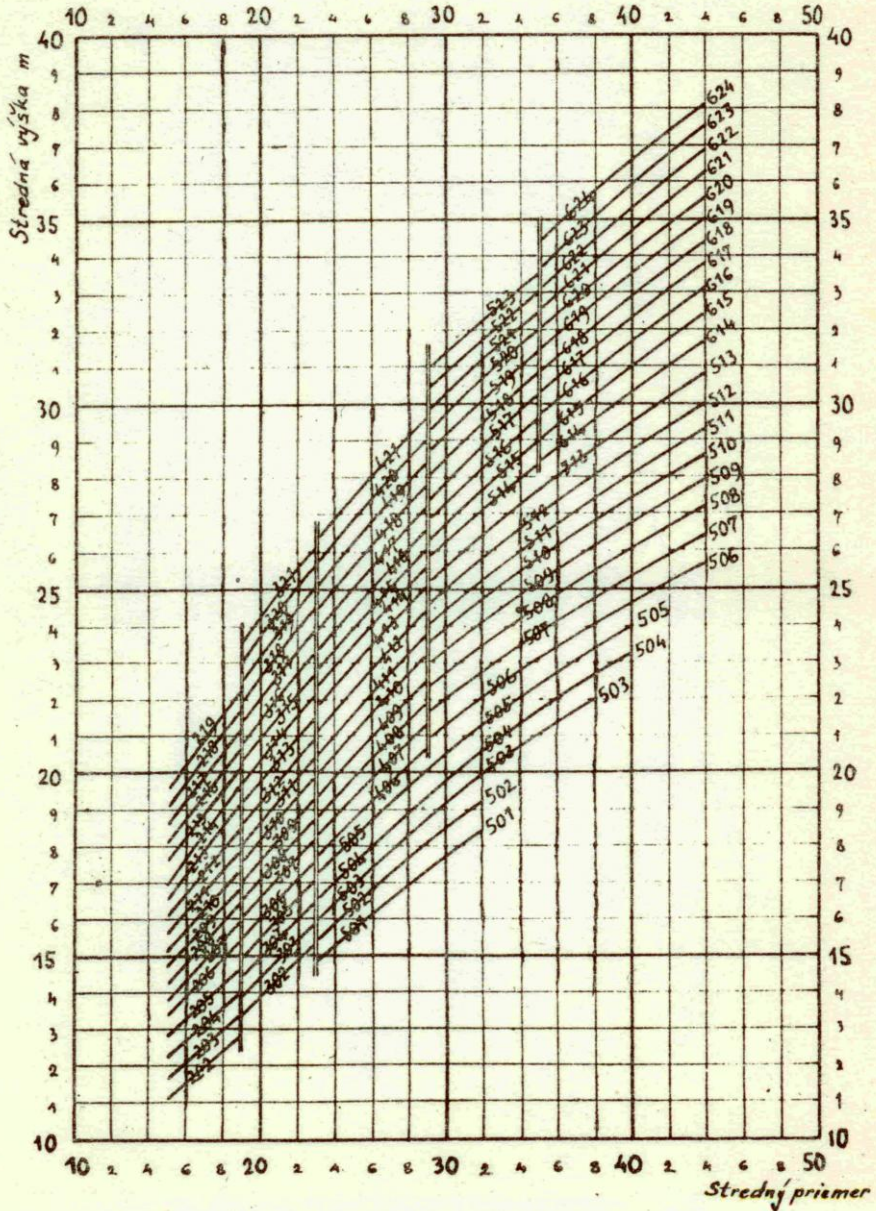
Grafikon pre určenie čísla JOK
