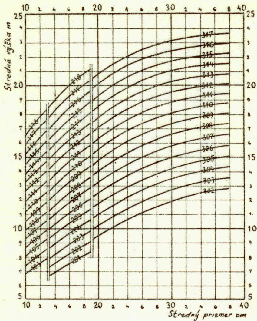
Grafikon pre určenie čísla JOK
