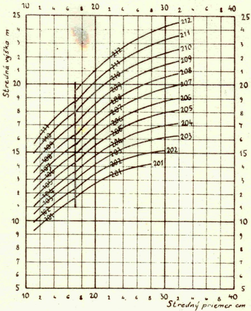
Grafikon pre určenie čísla JOK
