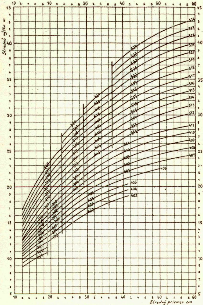
Grafikon pre určenie čísla JOK
