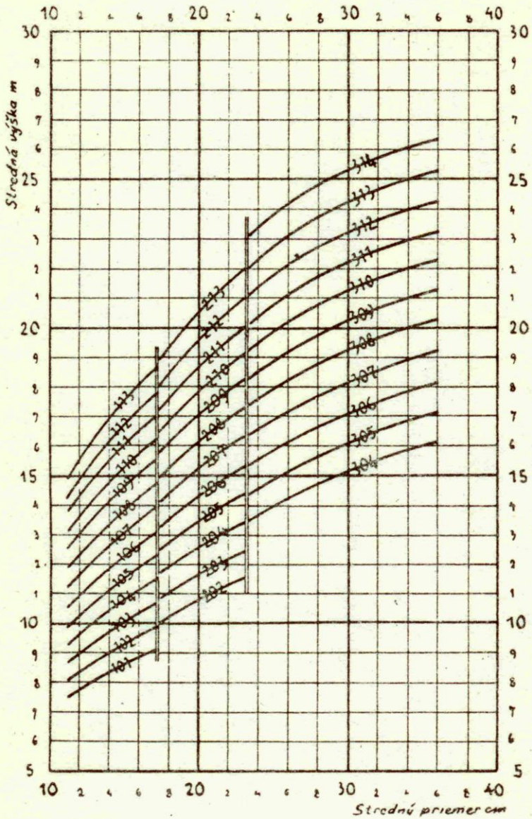
Grafikon pre určenie čísla JOK
