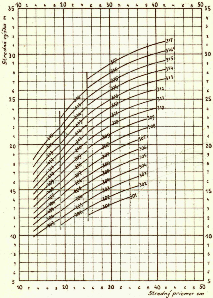
Grafikon pre určenie čísla JOK
