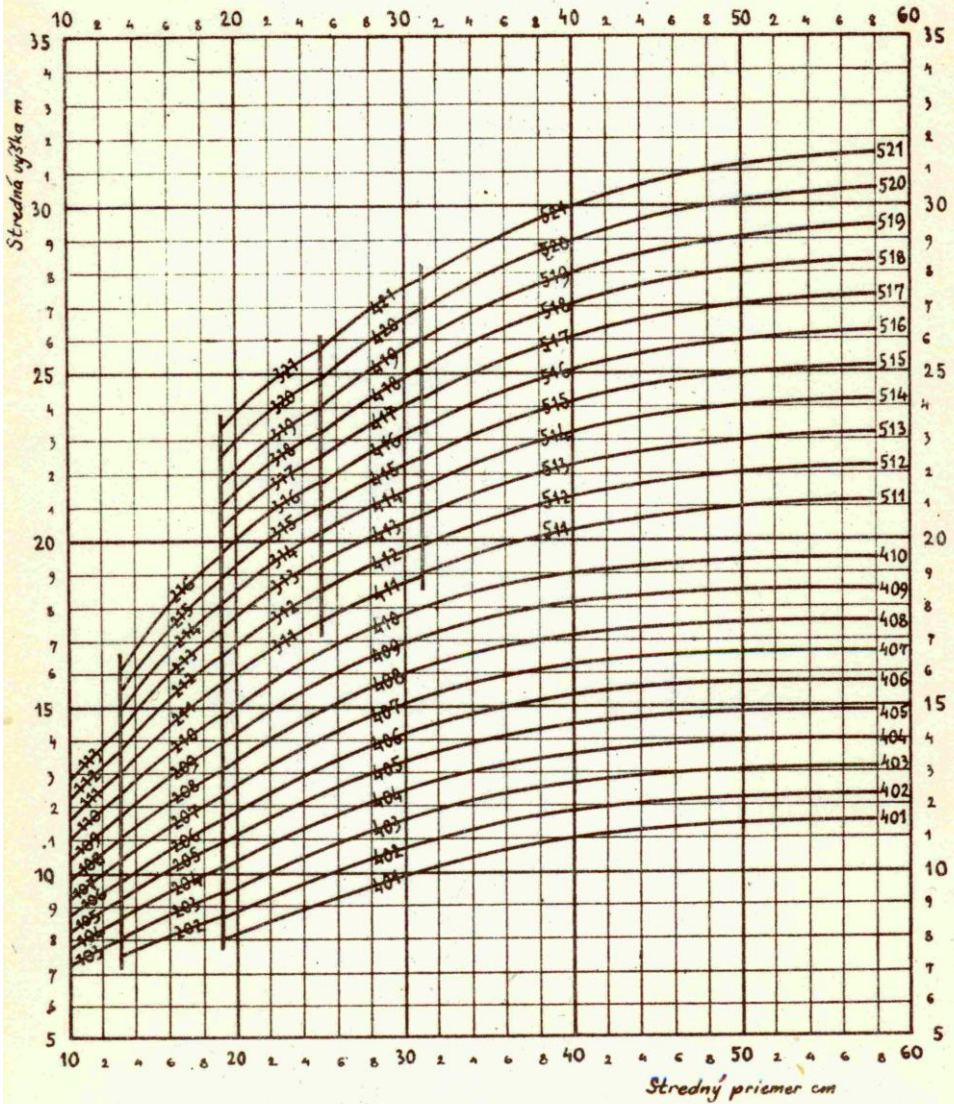
Grafikon pre určenie čísla JOK
